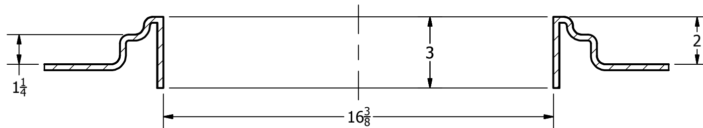
SECTION A-A SCALE 1:4
